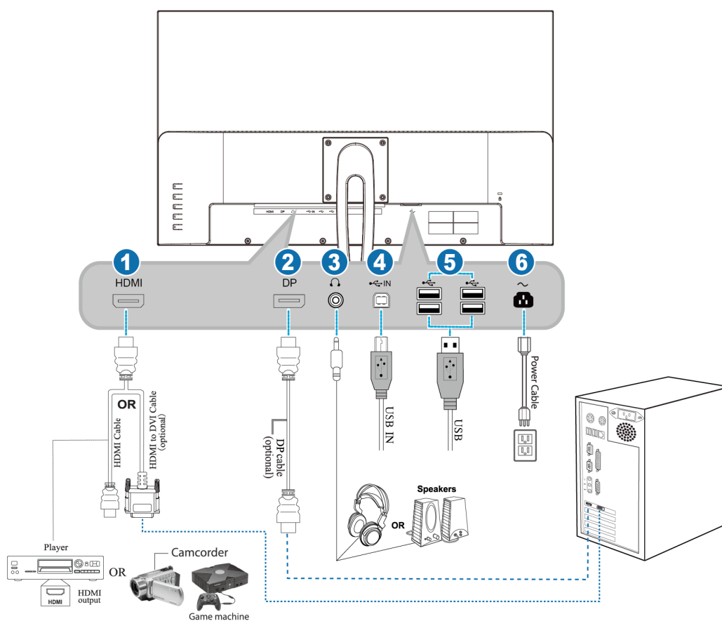
Figura 2. Conexión a un PC
